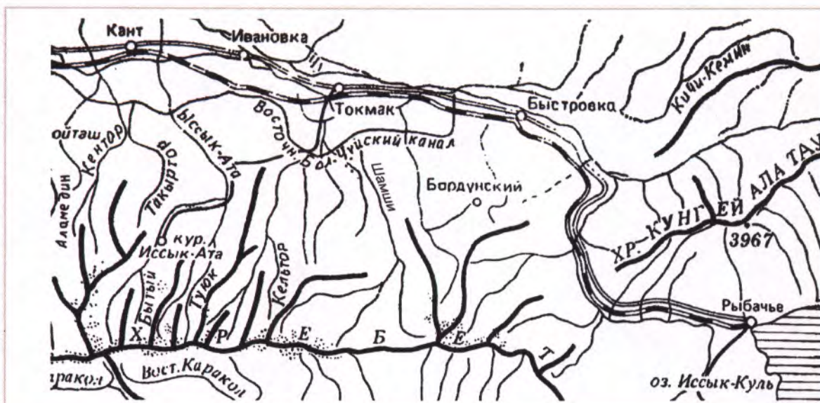
Орографическая схема восточной части Киргизского хребта
