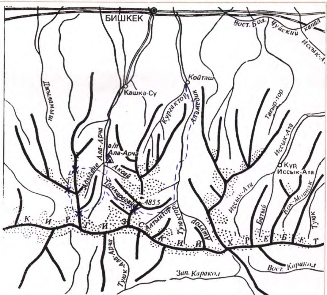
Орографическая схема центральной части Киргизского хребта
